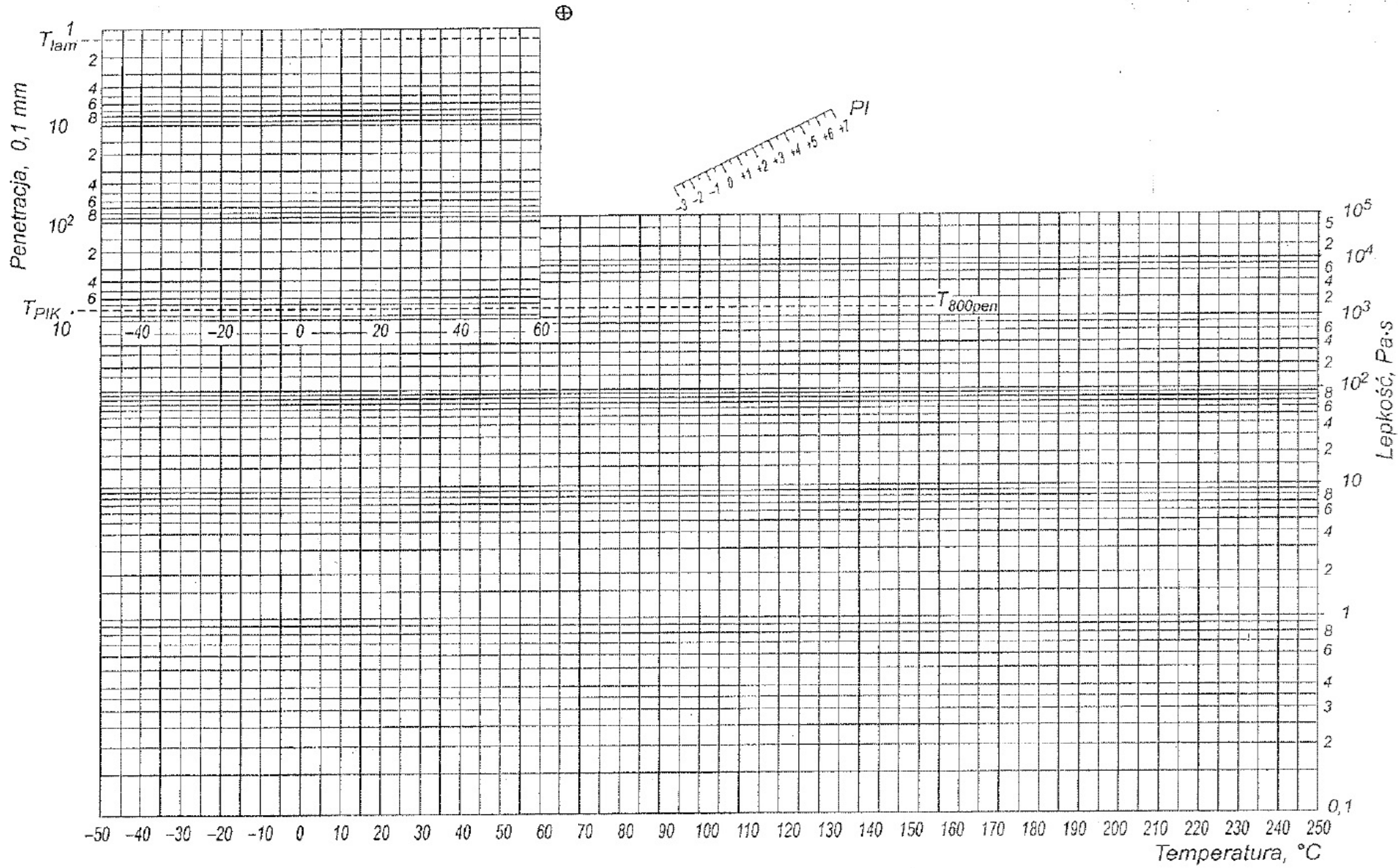
Karta Jakości Asfaltu. Wykres BTDC
